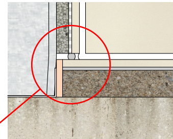
1 Vertical section Scale: 3" = 1'-0"
