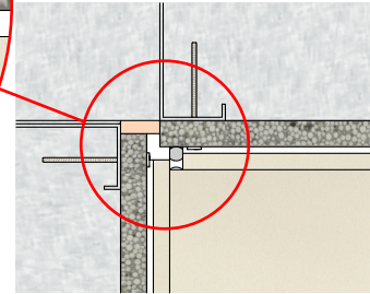
1 Horizontal section Scale: 3" = 1'-0"
