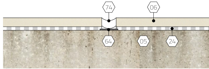
1 Section Scale: 6" = 1'-0"
