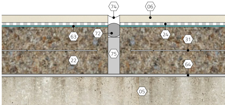
1 Section Scale: 6" = 1'-0"
