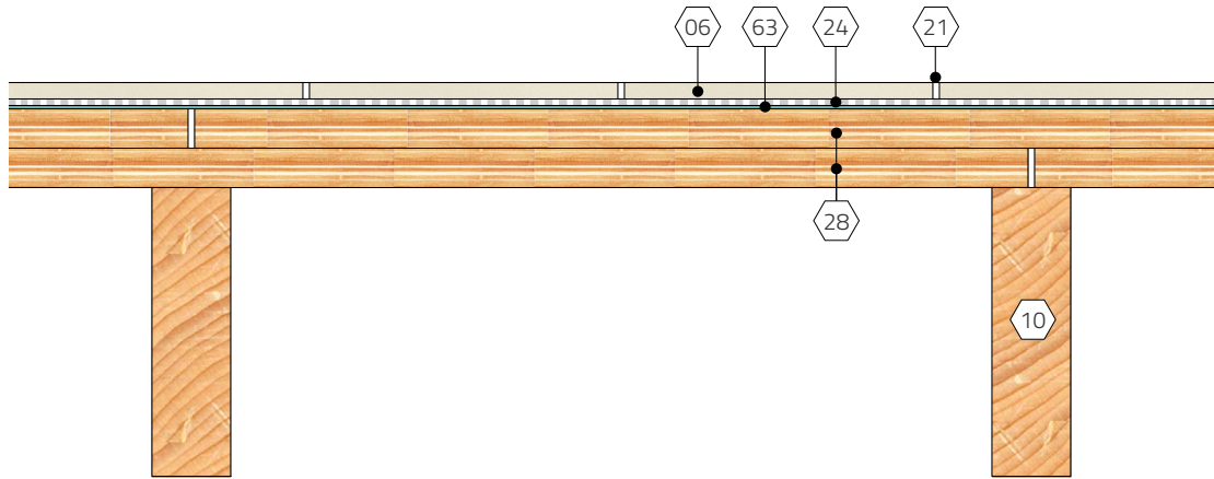
1 Section Scale: 3" = 1'-0"
