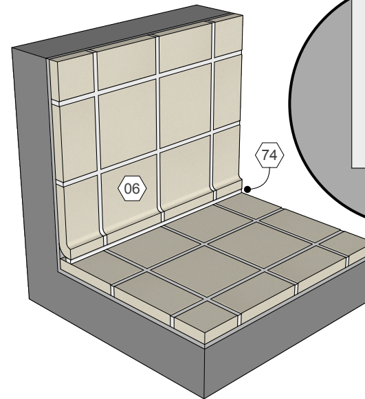
3 Cove base, thin lip Scale: N.T.S.
