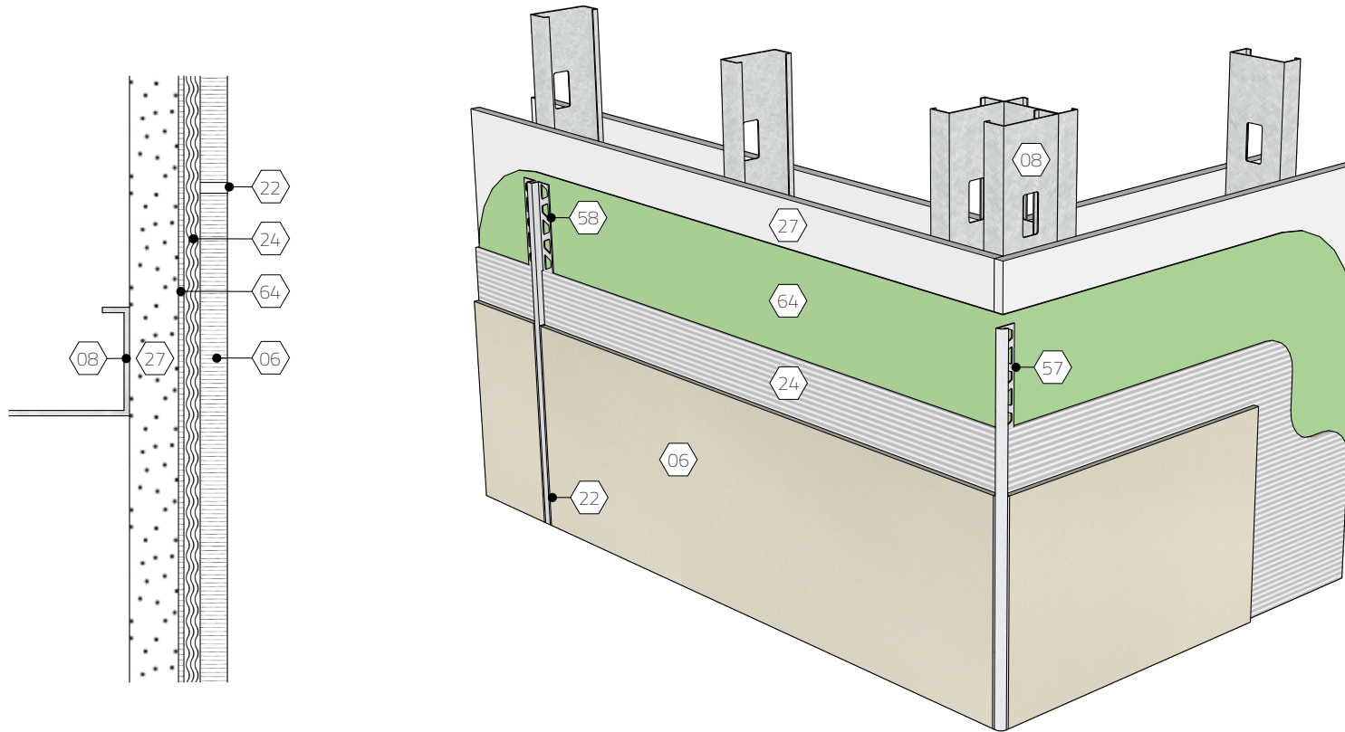
1 Section Scale: 6" = 1'-0"
