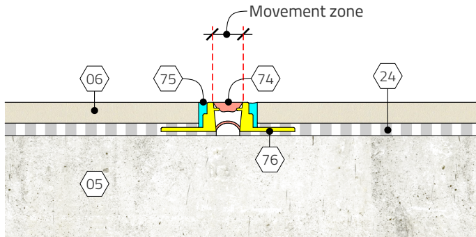
1 Section Scale: 6" = 1'-0"
