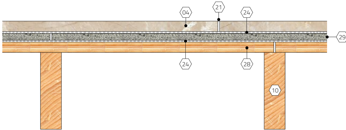
1 Section Scale: 3" = 1'-0"
