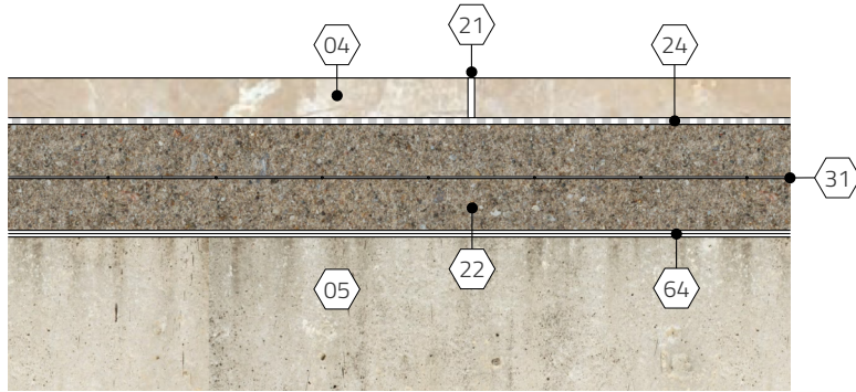
1 Section Scale: 3" = 1'-0"
