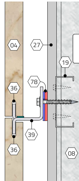
Section Scale: 3" = 1'-0"
