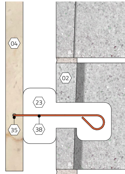
Section Scale: 3" = 1'-0"
