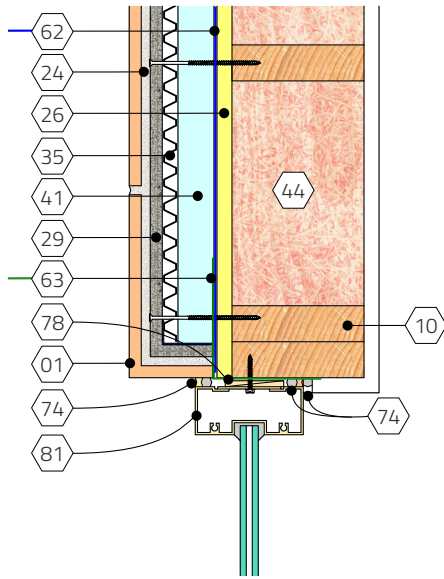
3 Jamb Scale: 1 1/2" = 1'-0"
