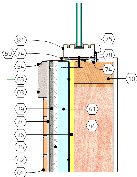
1 Sill Scale: 1 1/2" = 1'-0"
