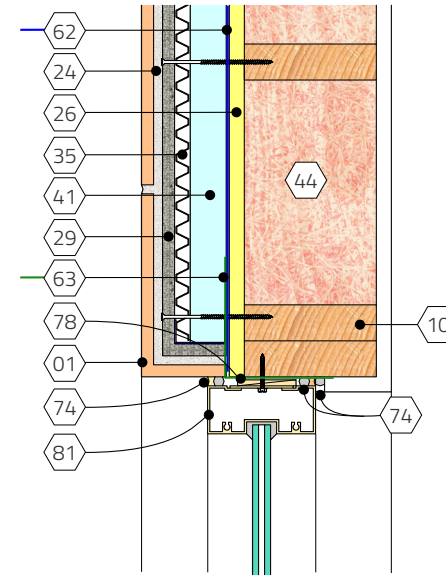
2 Jamb Scale: 1 1/2" = 1'-0"
