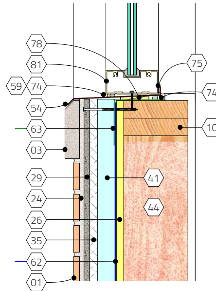
3 Sill Scale: 1 1/2" = 1'-0"
