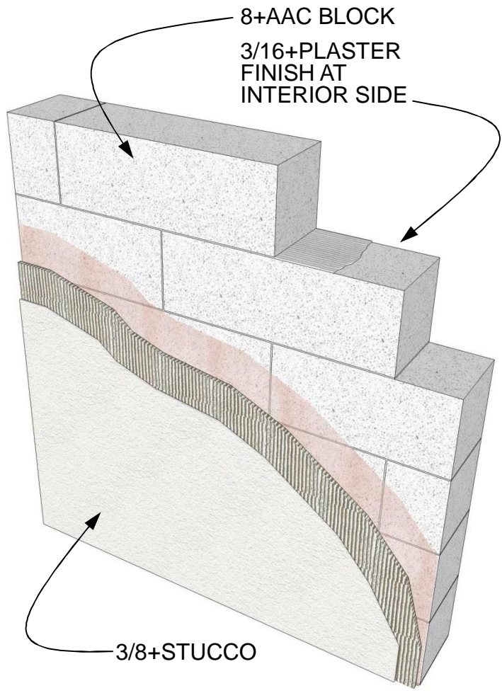
AAC Wall R=15.75
