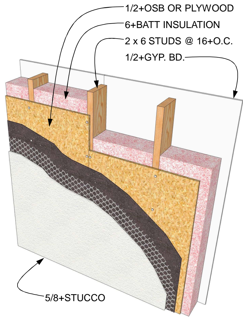
Wood Stud Wall R=15.75
